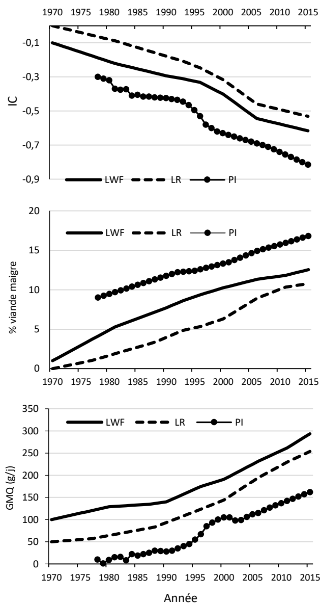
Figure 4 – Évolutions génétiques estimées pour le gain moyen quotidien (GMQ), l'indice de consommation (IC) et la teneur en viande maigre de la carcasse. LW : Large White femelle ; LR : Landrace Français ; PI : Piétrain. Les valeurs initiales pour chaque race sont fixées arbitrairement pour permettre de différencier les courbes
